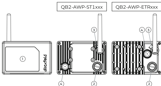
Figure 1 Vue d'ensemble du LiDAR.
