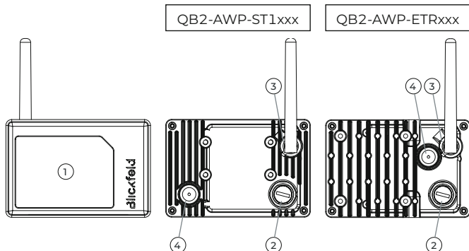
图1 LiDAR概览。LiDAR正面(左)、背面(中、右)。
